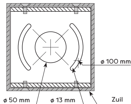
B-B doorsnede (afmetingen van positioneerbare voetplaat)
