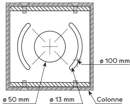
Section B-B (dimensions de la plaque de base positionnable)
