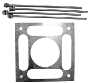
Moule de positionnement espacement de 200 x 200 mm
